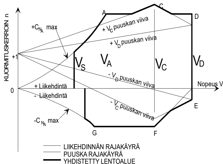
Kuva 1. Esimerkki lennon rajakäyrästä puuskasuorineen.
